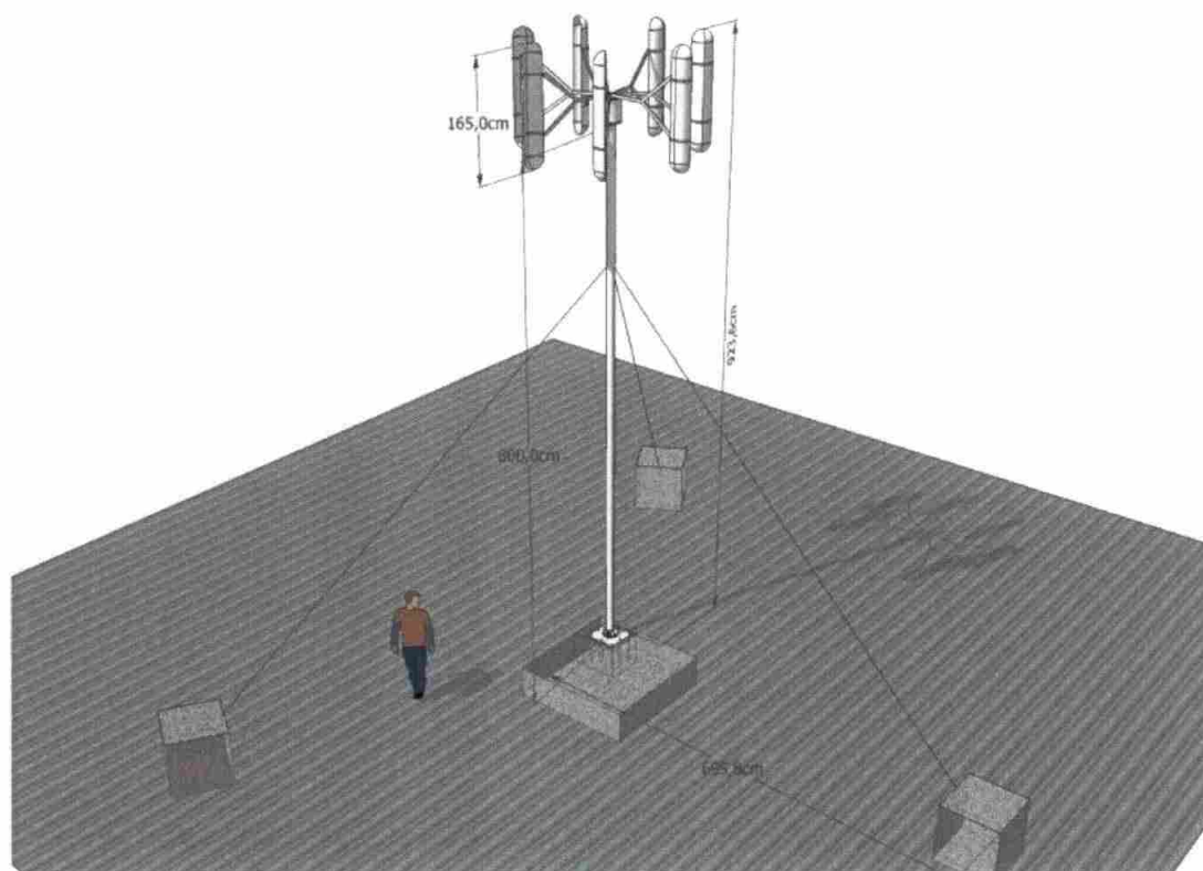
RYSUNEK 44: PARAMETRY TECHNICZNE MIKROTURBINY WIATROWEJ
