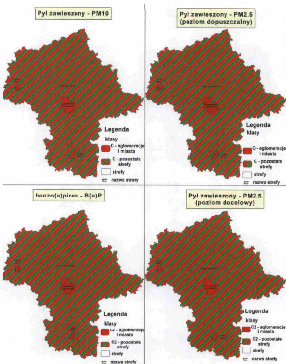
RYSUNEK 2: KLASYFIKACJA STREF WG ZANIECZYSZCZEN: PM10, PM2,5, B(A)P – OCHRONA ZDROWIA
