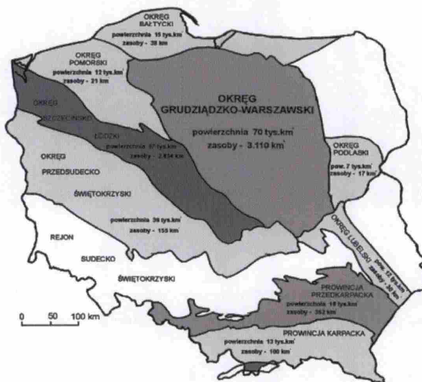
RYСУNEK 45: PROWINCJE I OKRĘGI GEOTERMALNE W POLSCE
