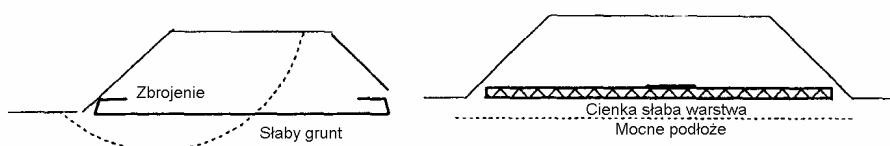
Rys. 2.2. Przykłady zbrojenia nasypów geosyntetykami
