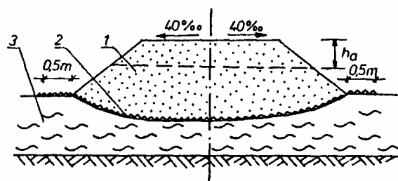
Rys. 2.1. Schemat nasypu na gruncie słabonośnym z zastosowaniem geosyntytyku 1 - nasyp drogowy, 2- warstwa geosyntytyku, 3 - grunt słabonośny
