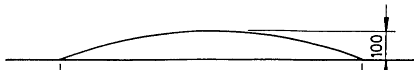
Rys. 1. Kształt i wymiary progów liniowych typu 1 (dla granicznej prędkości przejazdu 25-30 km/h) Próg listwowy typu 1
