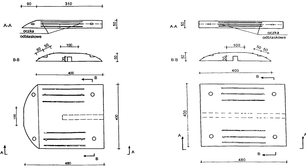
Rys. 3. Próg typu listwowego o długości 900 mm i wysokości 50 mm
