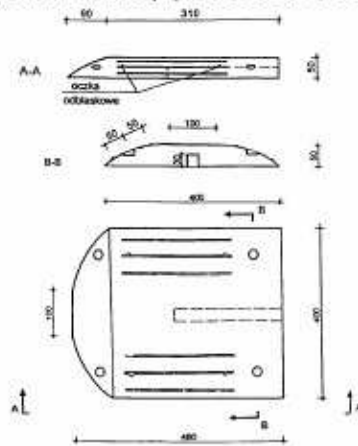
b) Element środkowy szerokości 480 mm
