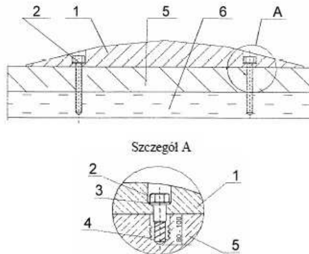
Rys. 4. Przykład umocowania progu do nawierzchni jezdni
