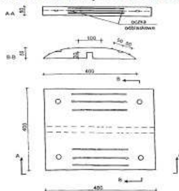
b) Element środkowy szerokości 480 mm
