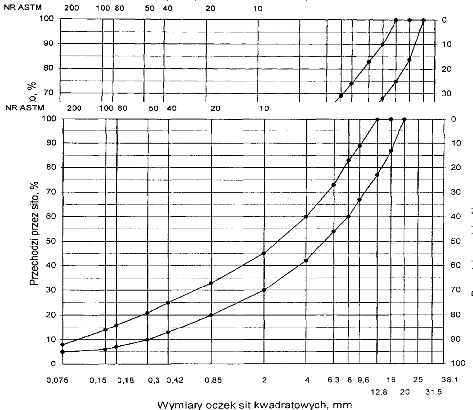
Rys. 12. Krzywe graniczne uziarnienia mieszanki mineralnej BA od 0 do 20 mm do warstwy wiążącej, wyrównawczej i wzmacniającej nawierzchni drogi o obciążeniu ruchem od
