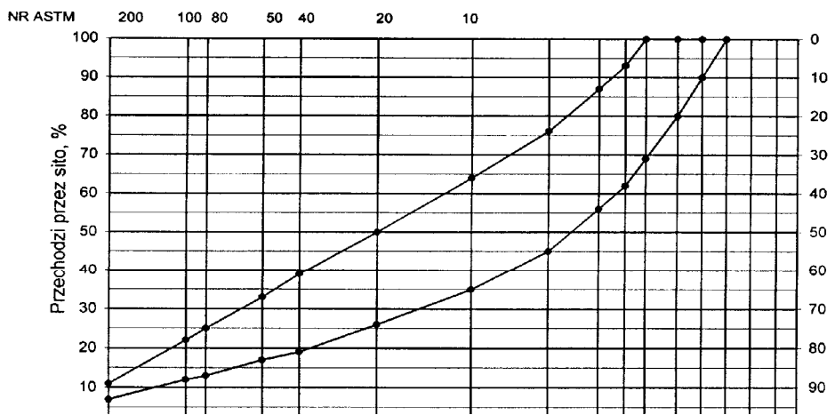
Rys. 2. Krzywe graniczne uziarnienia mieszanki mineralnej BA od 0 do 16mm, od 0 do 12,8 mm do warstwy ścieralnej nawierzchni drogi o obciążeniu ruchem KR1 lub KR2
