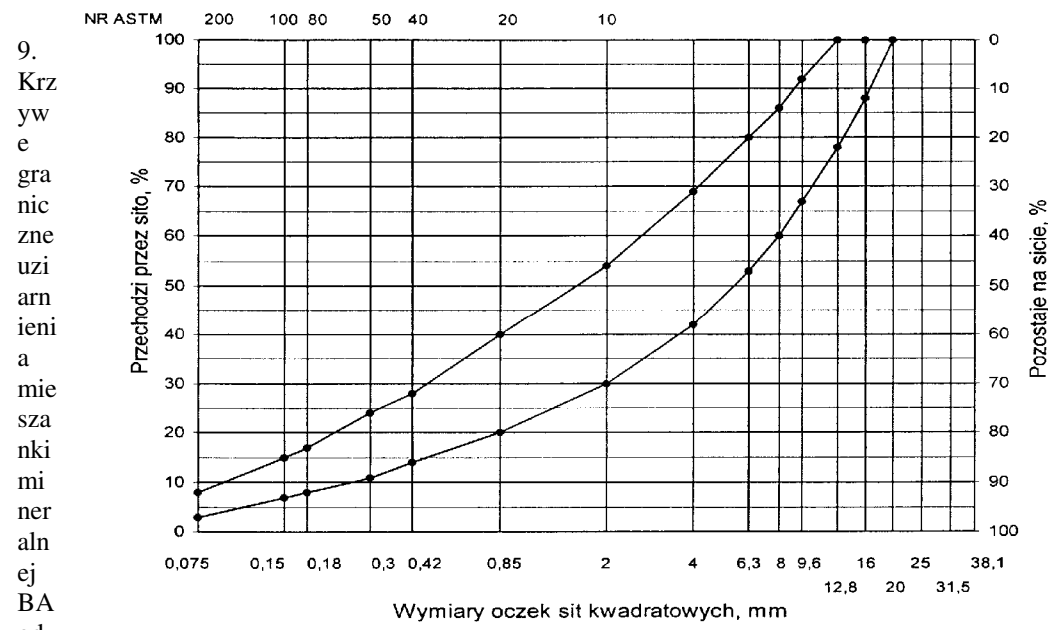
9. Krzywe graniczne uziarnienia mieszanki mineralnej BA od 0 do 16 mm do warstwy wiążącej, wyrównawczej i wzmacniającej nawierzchni drogi o obciążeniu ruchem KR1 lub KR2
