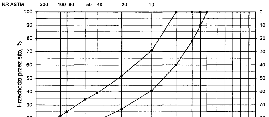
Rys. 3. Krzywe graniczne uziarnienia mieszanki mineralnej BA od 0 do 8mm, od 0 do 6,3 mm do warstwy ścieralnej nawierzchni drogi o obciążeniu ruchem nawierzchni drogi o obciążeniu ruchem KR1 lub KR2
