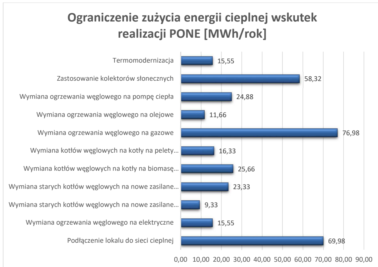
RYSUNEK 45 OGRANICZENIE ZUŻYCIA ENERGII CIEPŁEJ WSKUTEK REALIZACJI PONE [MWh/ROK].
