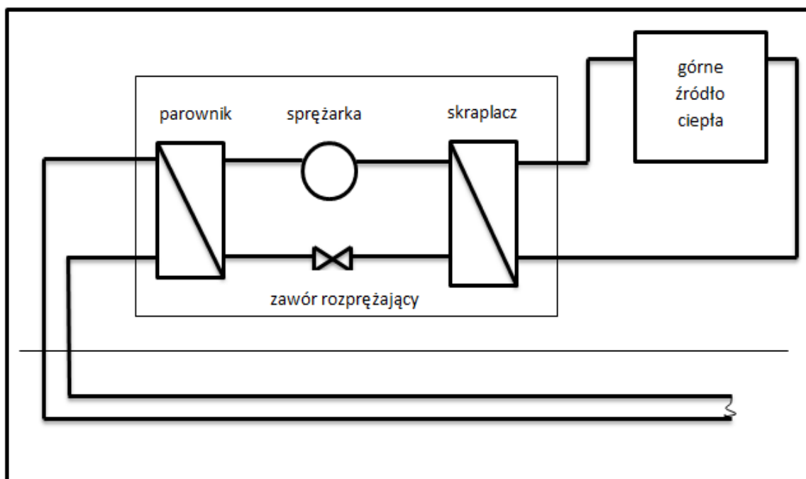
RYSUNEK 36: SCHEMAT DZIAŁANIA SPRĘŻARKOWYCH POMP CIEPŁA
