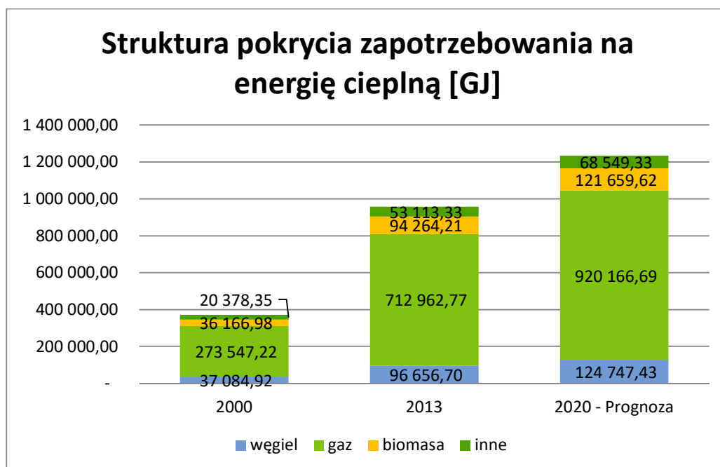
RYSUNEK 20: STRUKTURA POKRYCIA ZAPOTRZEBOWANIA NA ENERGIĘ CIEPLNĄ [GJ]
