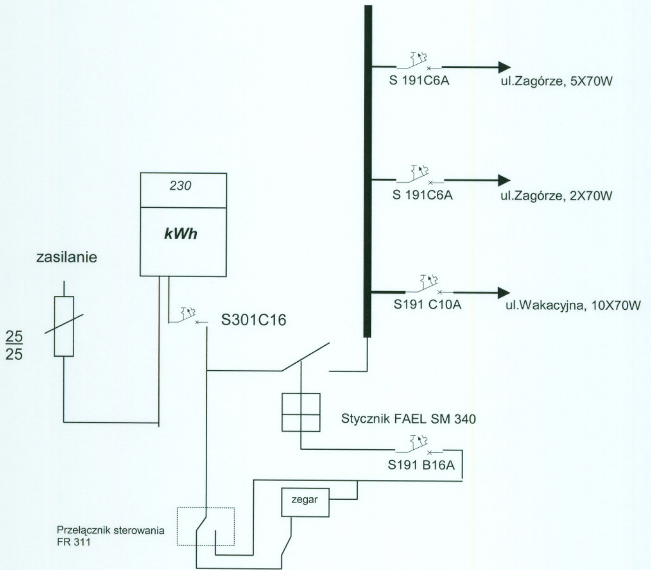
Schemat jednokreskowy szafy oświetleniowej OS Zagórze r.Wakacyjnej.
