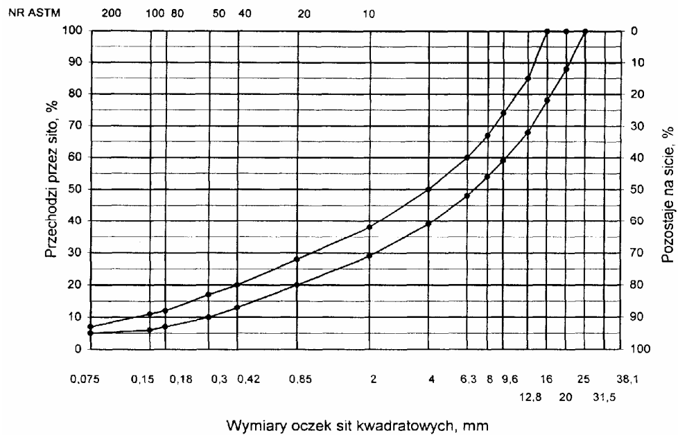
Rys. 4. Krzywe graniczne uziarnienia mieszanki mineralnej BA od 0 do 20 mm do warstwy ściaralnej nawierzchni drogi o obciążeniu ruchem od KR3 do KR6
