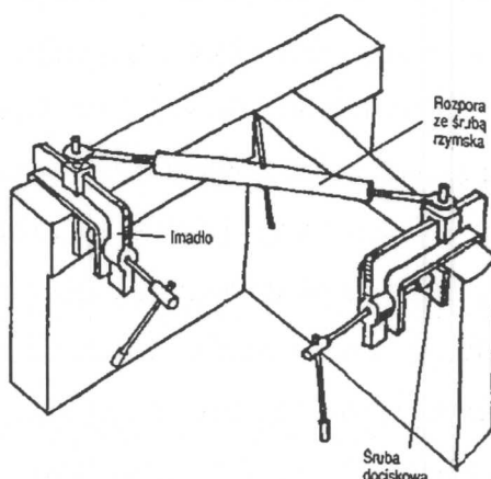
Rys. Przyrząd rozpierająco - ściągający
