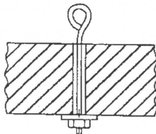
Rys. Uchwyt do demontażu wielkopłytowych płyt stropowych
