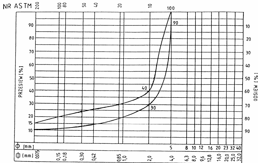
Rys. 1. Krzywe graniczne uziarnienia mieszank mineralnych SMA od 0 mm do 4 mm
