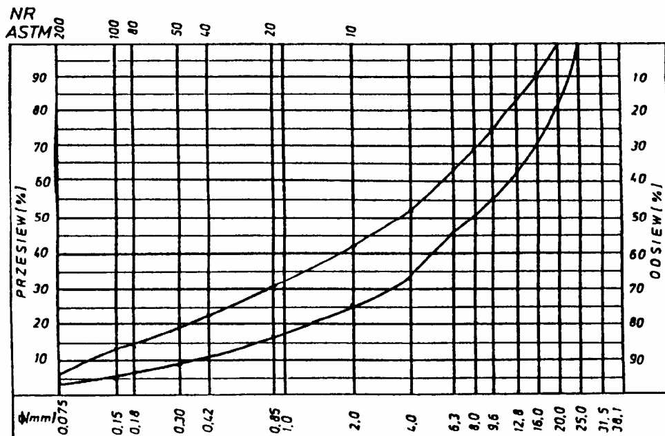
Rys. 2. Krzywe graniczne uziarnienia mieszanki mineralnej 0+20 mm do warstwy wiążącej, wyrównawczej i wzmacniającej z betonu asfaltowego dla KR 3-6
