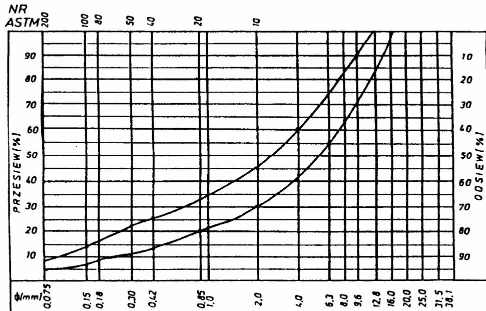
Rys. 3. Krzywe graniczne uziarnienia mieszanki mineralnej 0+16 mm do warstwy wiążącej, wyrównawczej i wzmacniającej z betonu asfaltowego dla KR 3-6
