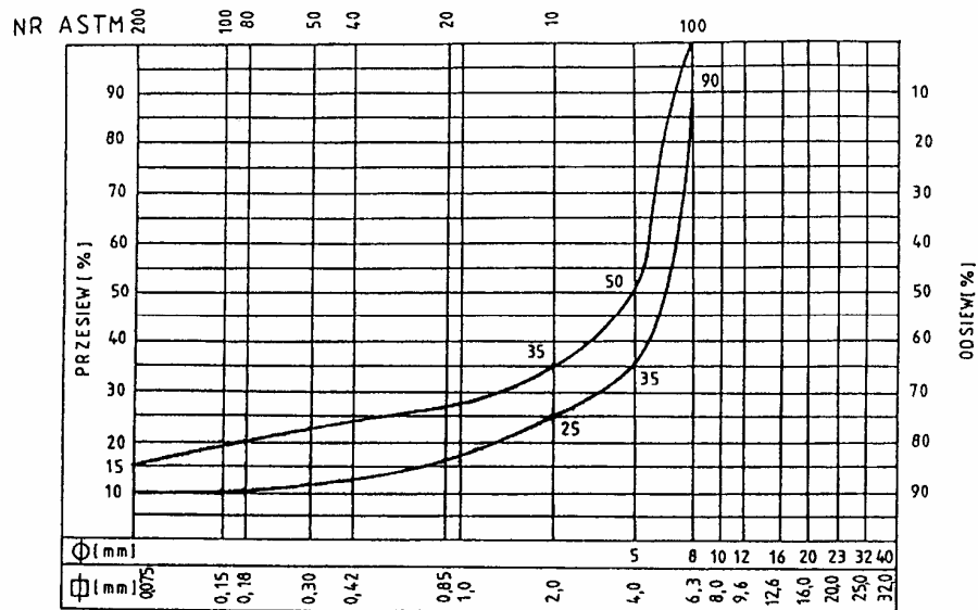
Rys. 2. Krzywe graniczne uziarnienia mieszank mineralnych SMA od 0 mm do 6,3 mm
