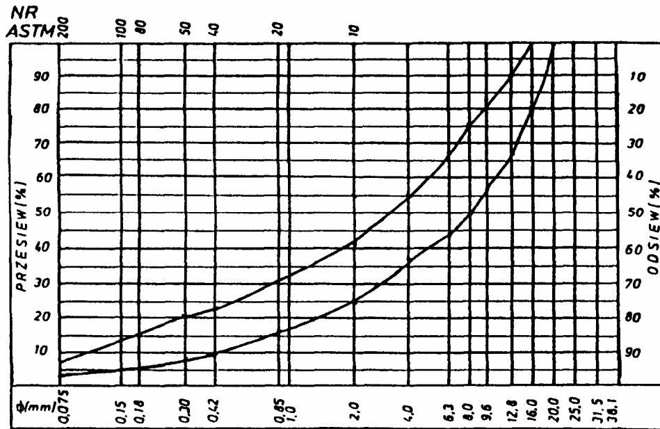
Rys. 1. Krzywe graniczne uziarnienia mieszanki mineralnej 0+25 mm do warstwy wiążącej, wyrównawczej i wzmacniającej z betonu asfaltowego dla KR 3-6
