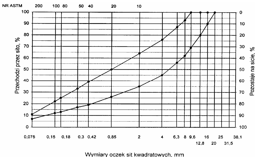
Rys. 2. Krzywe graniczne uziarnienia mieszanki mineralnej BA od 0 do 16mm, od 0 do 12,8 mm P.H.U. „DROG-POL II” sc Poświętne ul. Podmiejska 7, 09-100 Płońsk
