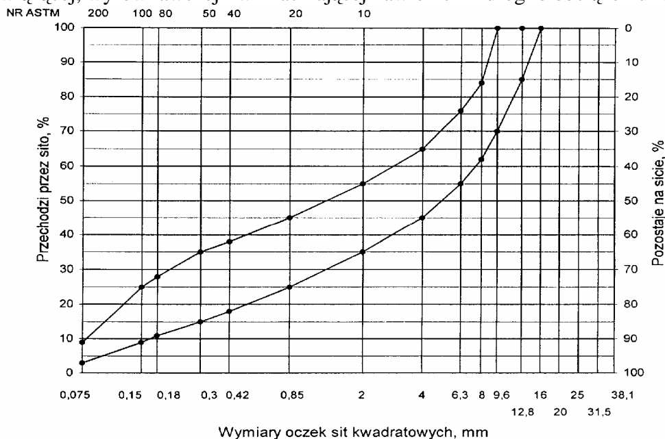
Rys. 6. Krzywe graniczne uziarnienia mieszanki mineralnej BA od 0 do 16 mm do warstwy wiążącej, wyrównawczej i wzmacniającej nawierzchni drogi o obciążeniu ruchem KR1 lub KR2
